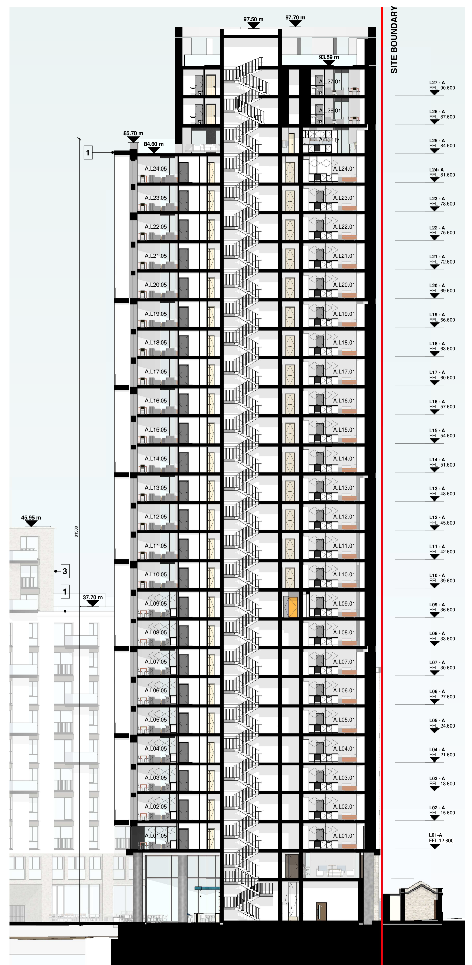
Section 4 - 4 1 : 200
