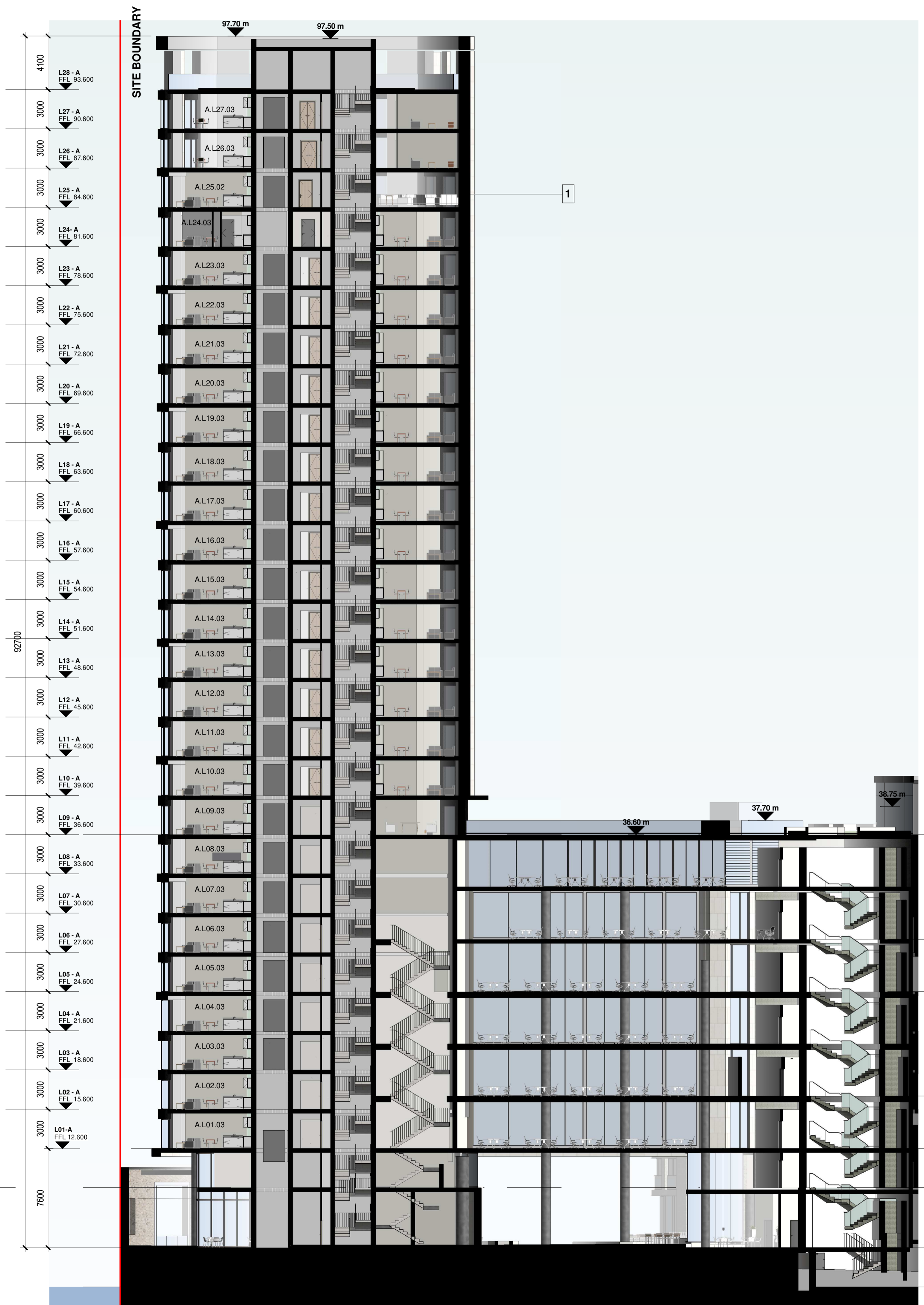
Section 3 - 3 1 : 200
